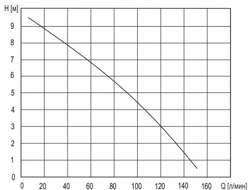
Рис. 1. Гидравлические характеристики.
