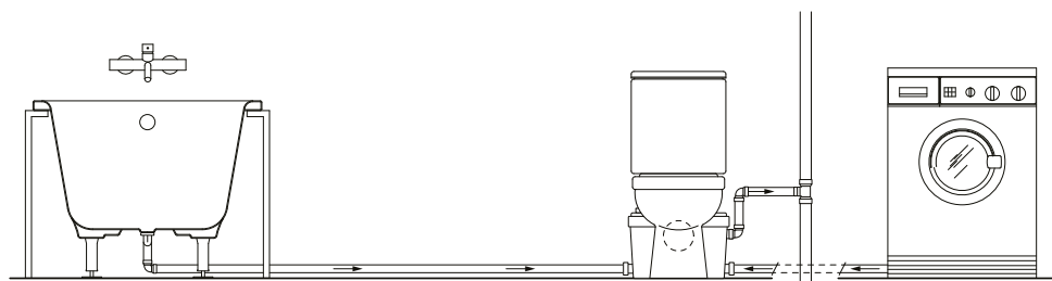
Рис. 3. Вариант подключения.
