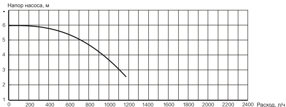
Стандартный водяной насос на 6 метров (L1PB20/26/30-RC1)
