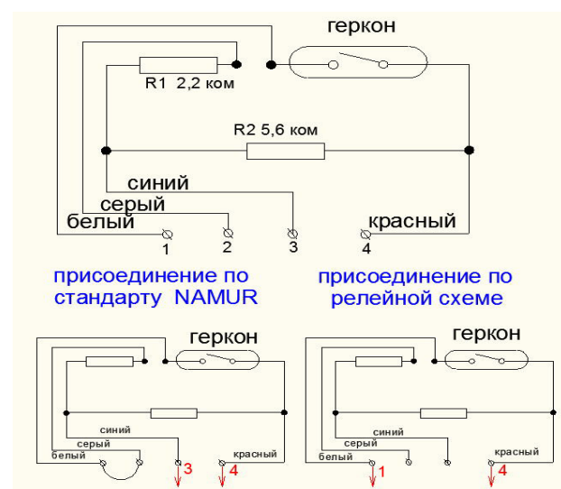
Рисунок 3. Схема импульсного выхода.
