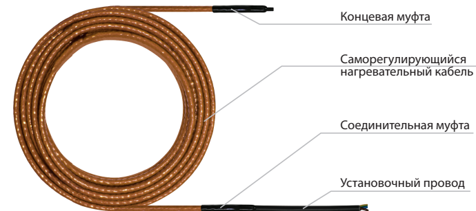
Рис. 1. Конструкция нагревательной секции
