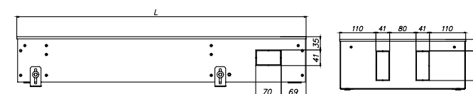
ЕКН.380.200, вид сбоку
