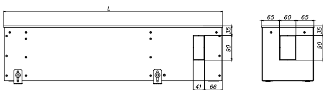
EKN.190.200, вид сбоку
