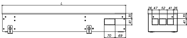
EKN.190.150 и EKN.190.200, вид сверху
