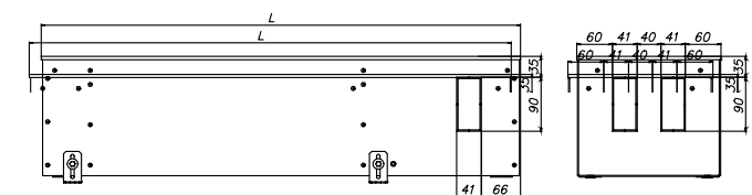
EKN.240.200, вид сбоку
