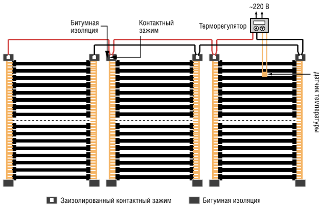
Рис. Общая схема подключения термопленки CALEO
