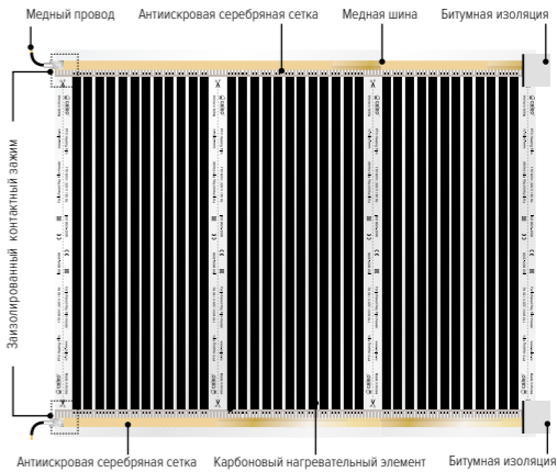
Рис. Общий вид термопленки CALEO, расположение основных ее элементов, контактных зажимов и мест подключения и изоляции
