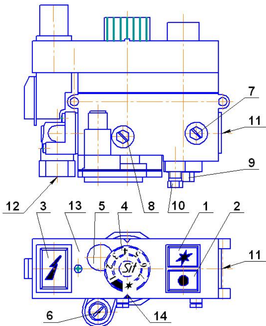
Рис.4 Элементы управления и регулировки газового клапана
