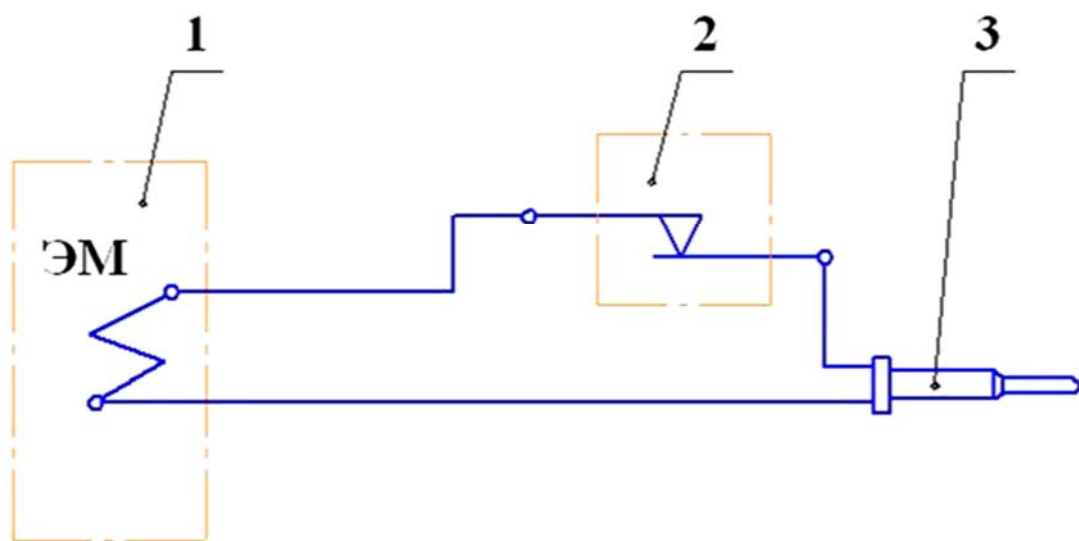
Рис.3 Схема электрическая.
