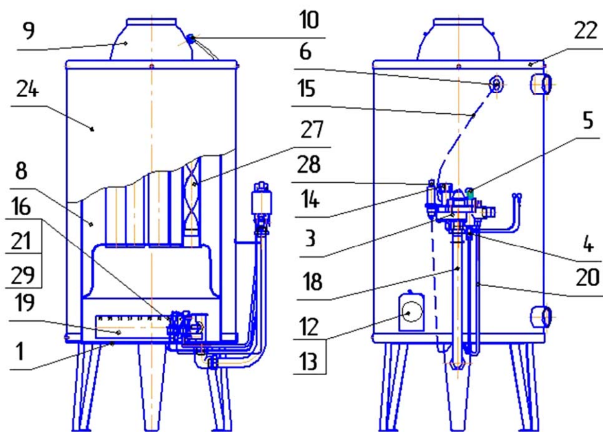
Рис.1 Конструкция аппарата.
